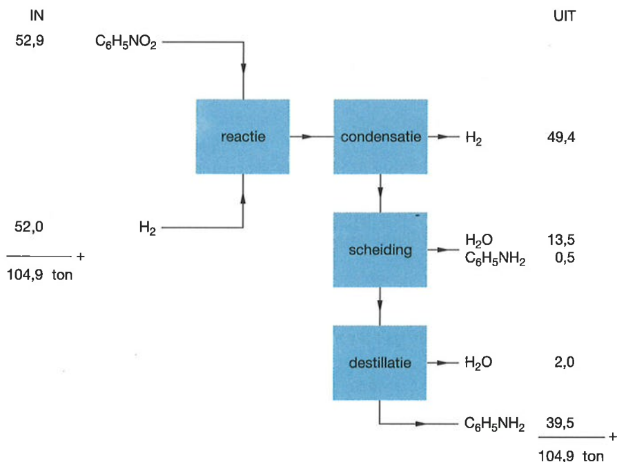
Proces 2: blokschema zonder recirculeren
