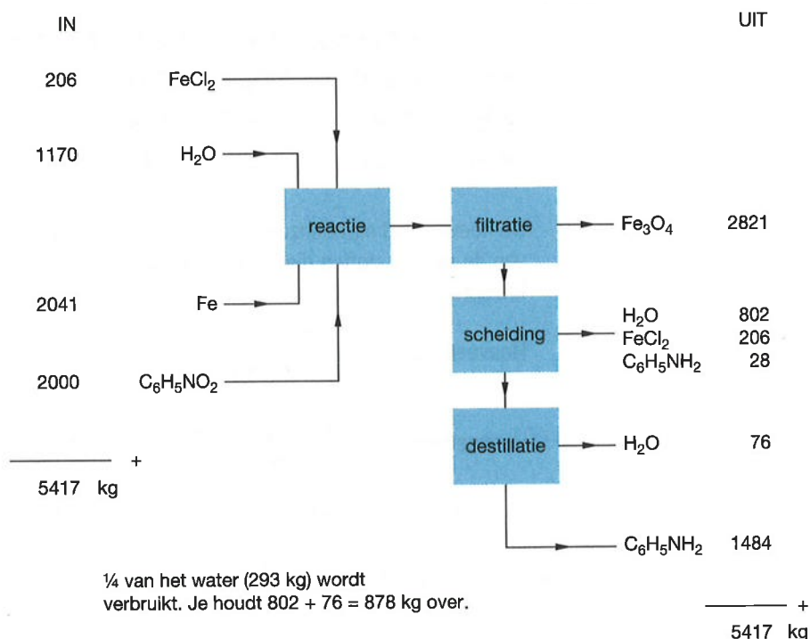
Proces 1: blokschema zonder recirculeren
