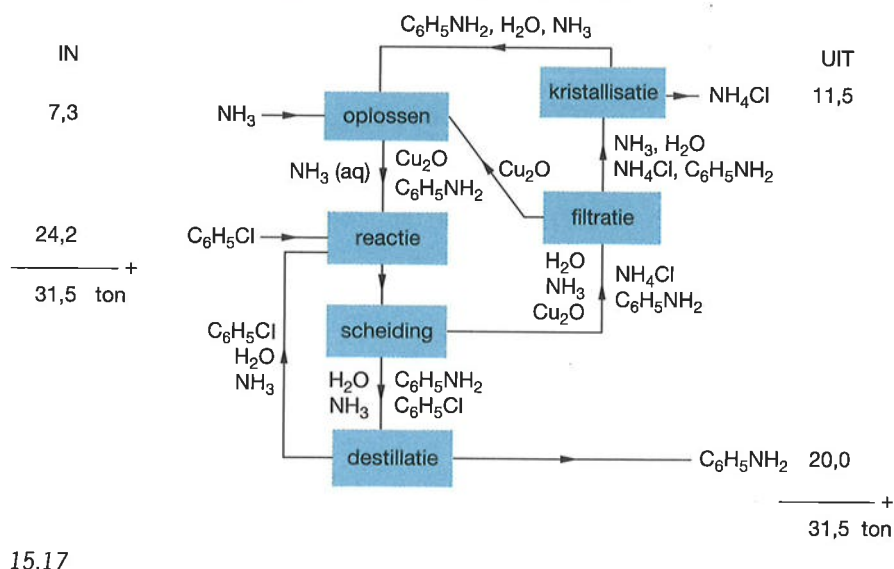
Proces 3: blokschema met recirculeren
