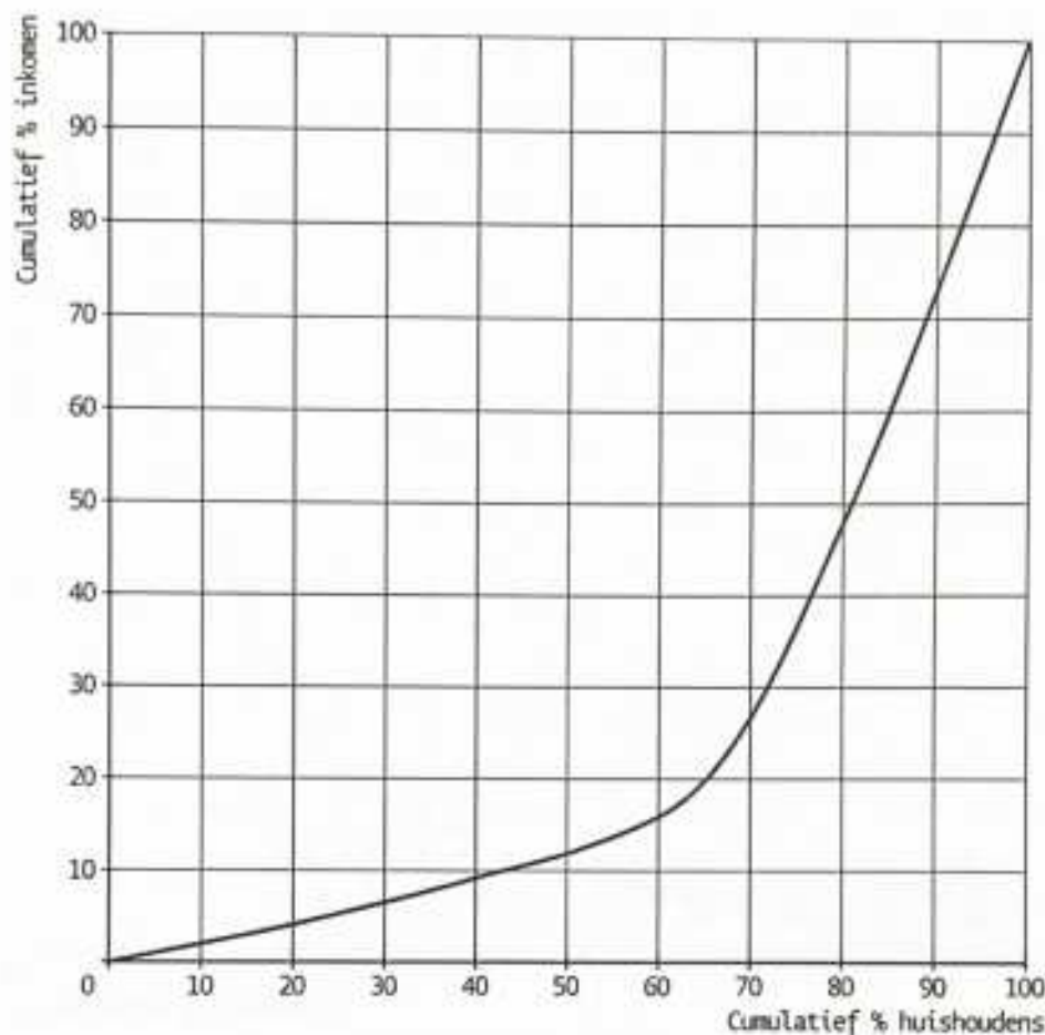
Lorenzcurve huishoudens
