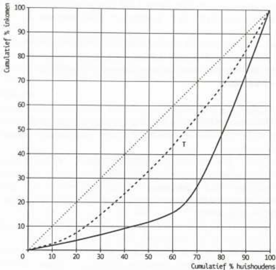
Lorenzcurve huishoudens
