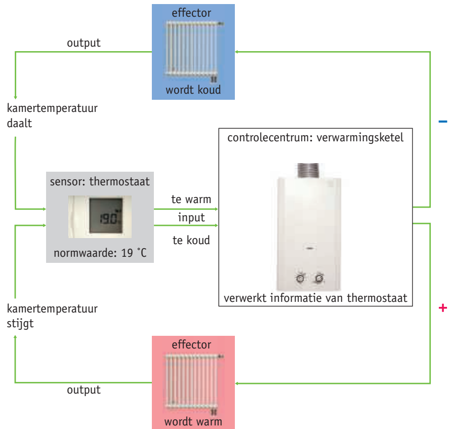
► Afb. 1 Een voorbeeld van een regelkring: het verwarmingssysteem in een huis.
