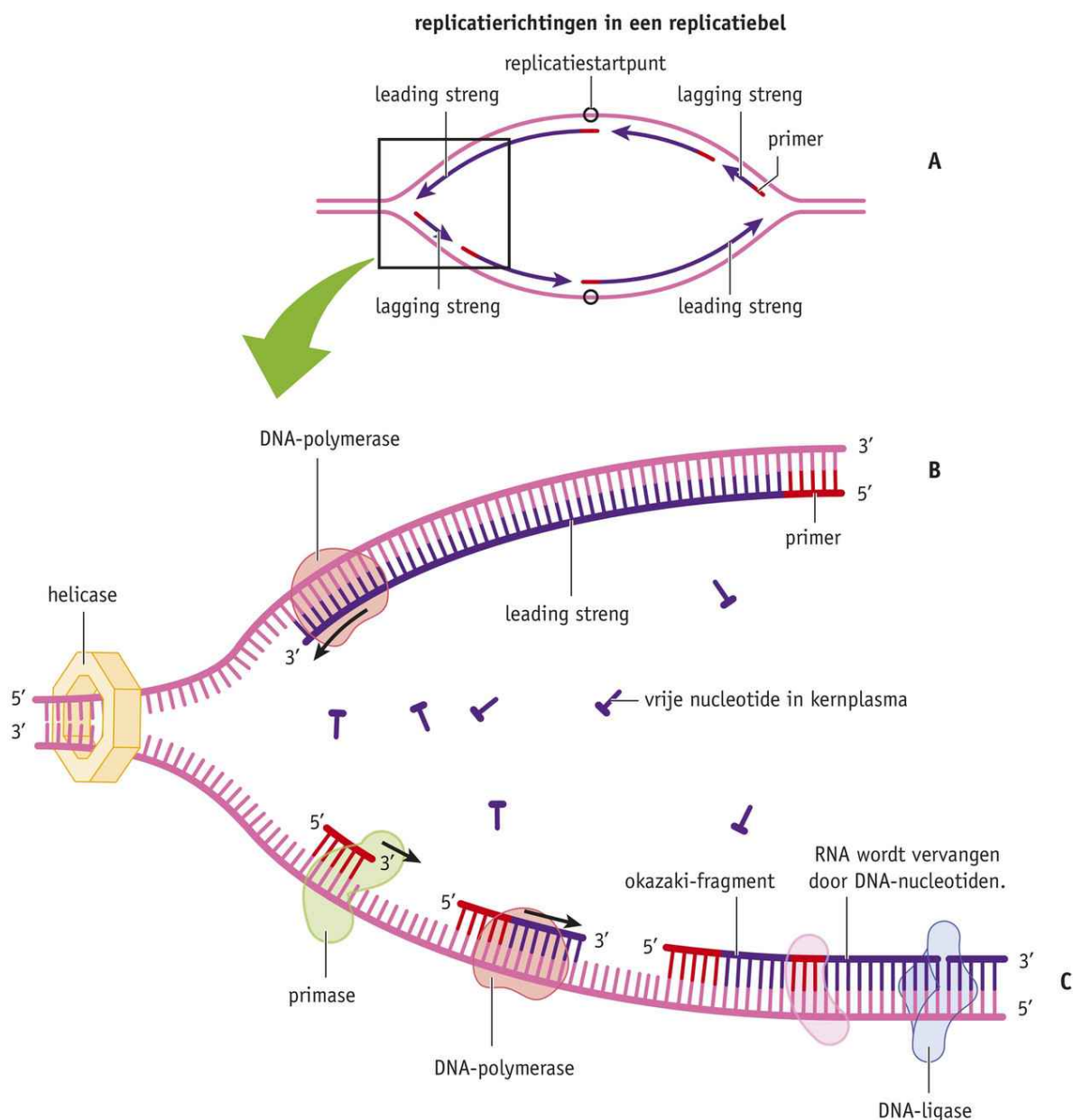
■ Afb. 12 DNA-replicatie.
