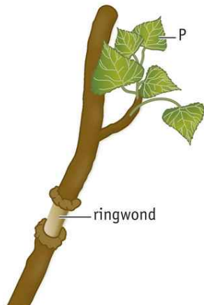
■ Afb. 23 Ringwondproef.
