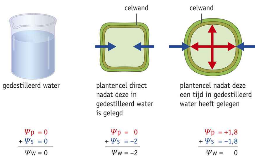
■ Afb. 16 Waterpotentiaal.
