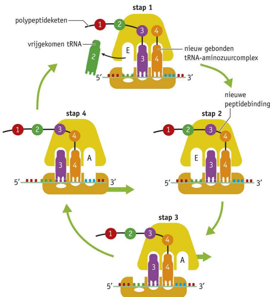
■ Afb. 38 Translatie.
