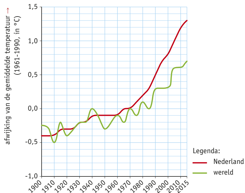
► Afb. 34 Verandering van de gemiddelde temperatuur in Nederland en in de wereld.
