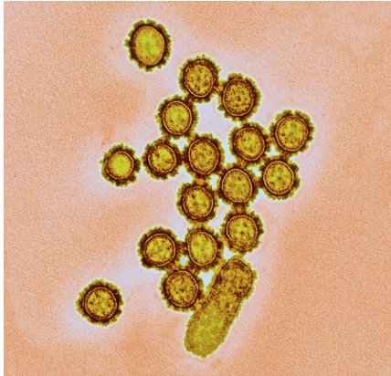
1 TEM
