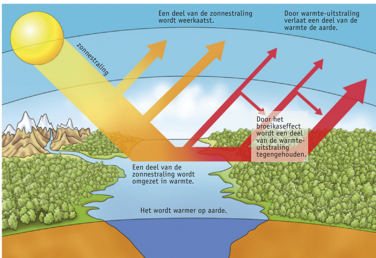
▼ Afb. 31 Het broeikaseffect.
