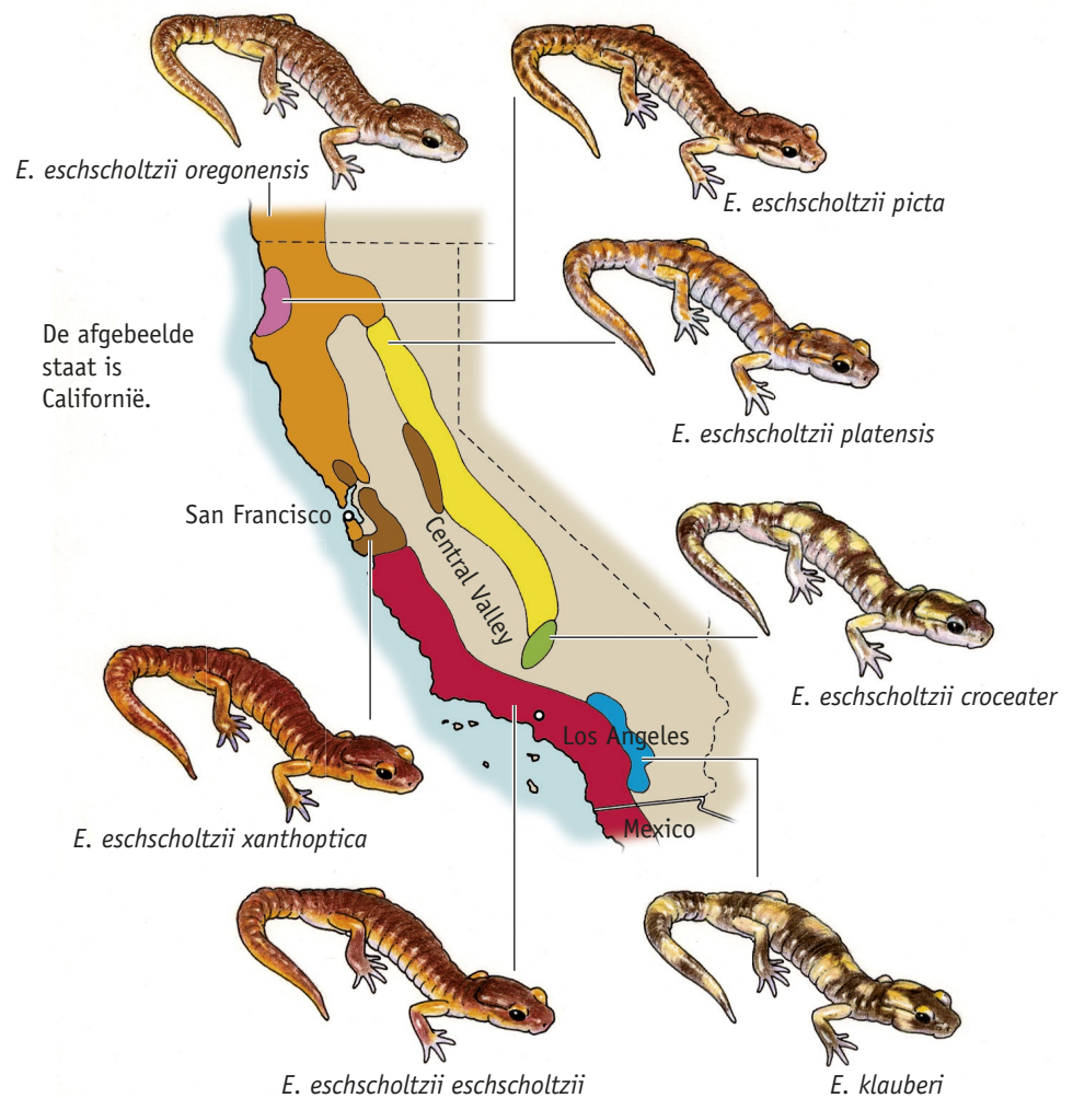
► Afb. 51 Leefgebied van Ensatina eschscholtzii en Ensatina klauberi .
