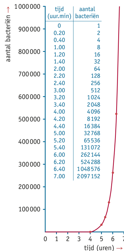
► Afb. 15 Exponentiële groei van bacteriën op een voedingsbodem.
