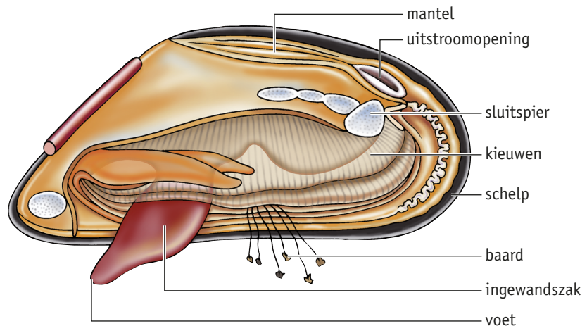
▼ Afb. 3 Inwendige bouw van de mossel (schematisch).
