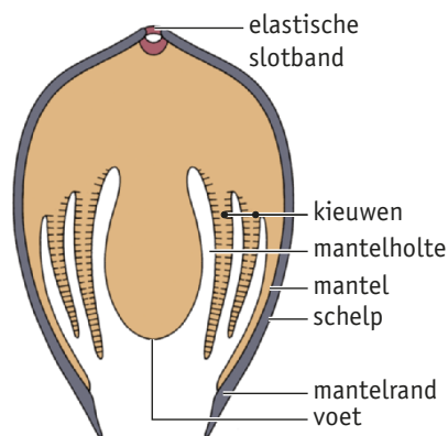
▼ Afb. 2 Mossel met weggeknipte mantel (schematisch).
