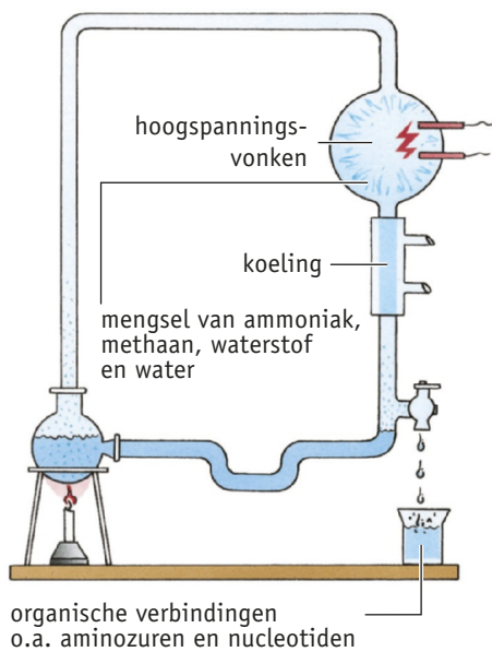
▼ Afb. 4 Toestel van Miller-Urey (schematisch).
