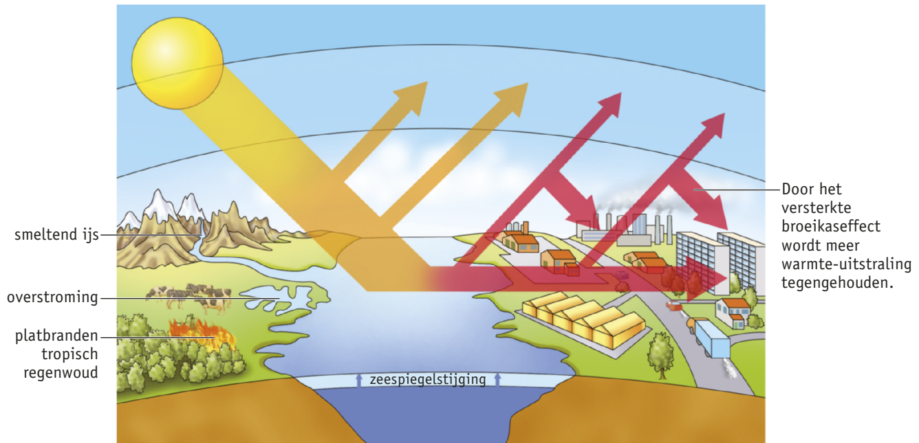
▼ Afb. 32 Het versterkte broeikaseffect.
