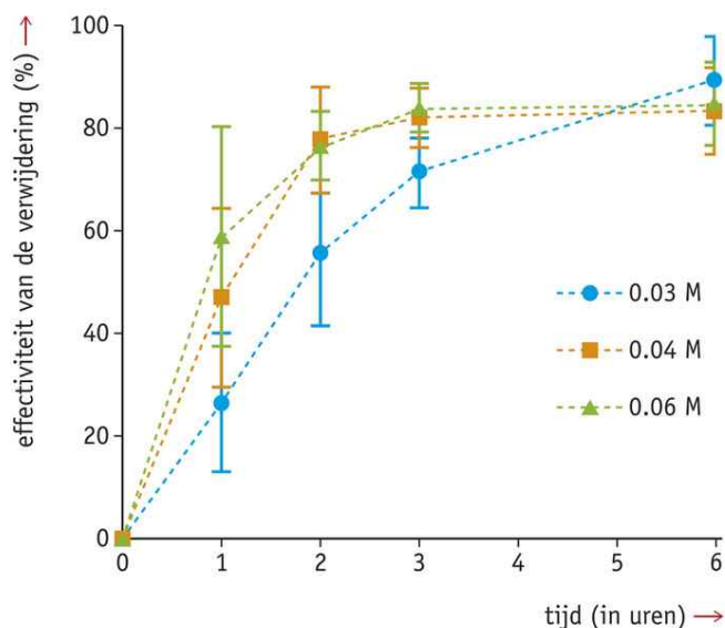
■ Afb. 70 Resultaten van het afbreken van microplastics met elektriciteit.
