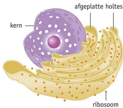
1 schematische tekening
