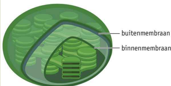
2 schematische tekening
