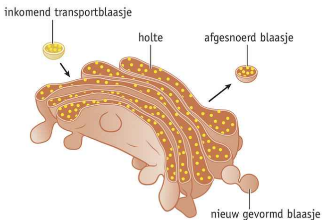
1 schematische tekening
