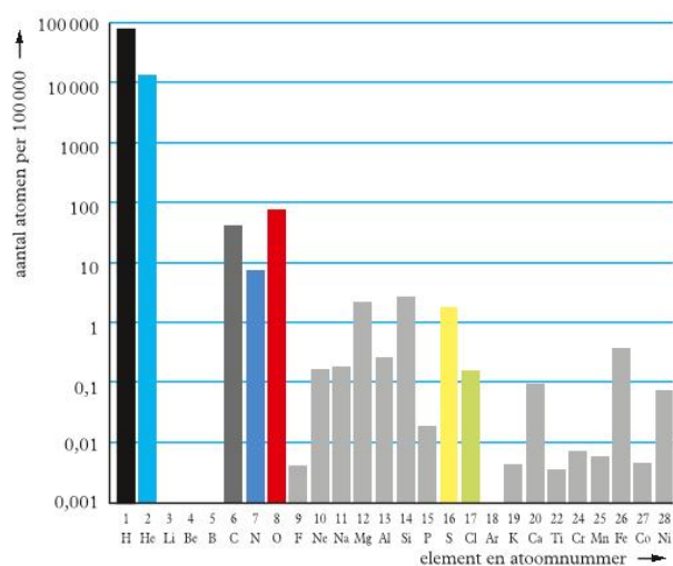
zon
