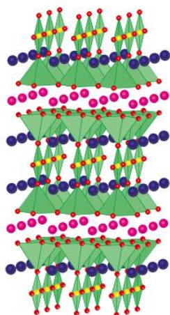
kubisch
